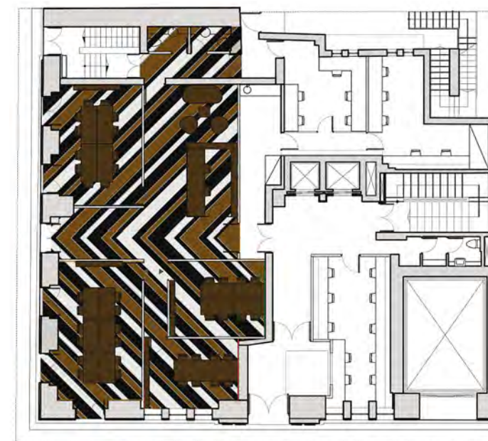
ΚΑΤΩΦΗ ΙΣΟΓΕΙΟΥ
